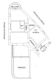
PLANIMETRIA ABITAZIONE PIANO QUINTO Hm= 3.55 m
