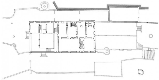
Villa Montefiano Pianta del primo piano Scala 1:200
