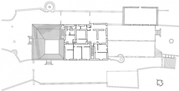
Villa Montefiano Secondo piano Scala 1:200
