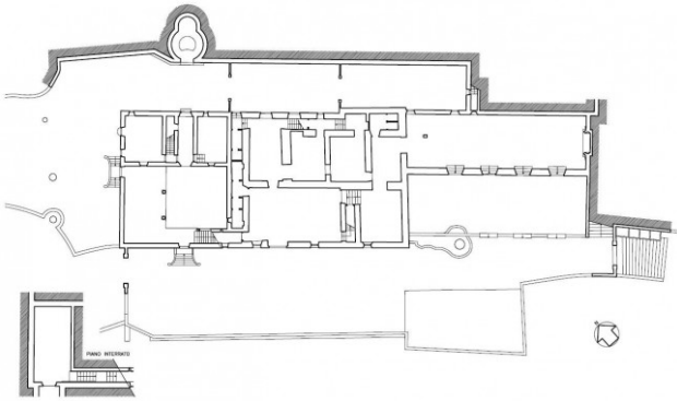
Villa Montefiano Pianta del piano terra Scala 1:200
