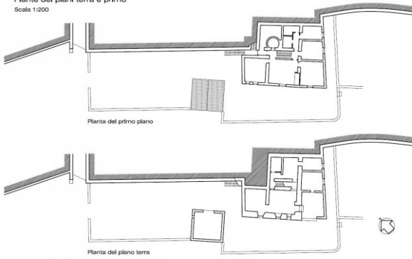
Casa colonica Fiano Pianta del piano terra e primo Scala 1:200
