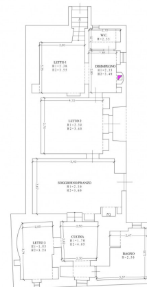
PIANTA PIANO TERRA (CORPO B) PROGETTO SCALA 1:100
