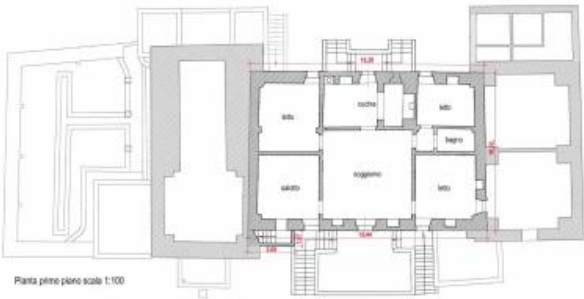
Pianta primo piano scale 1:100
