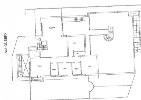
PIANO RIALZATO H= 3,05
