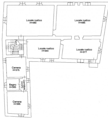
PIANO PRIMO
