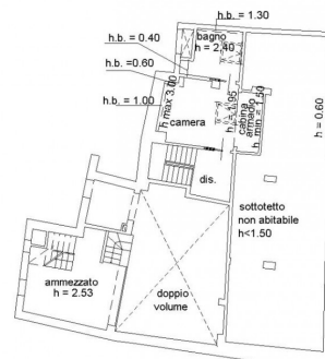
AMMEZZATO AL PIANO SECONDO E PIANO TERZO
