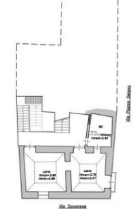
Pianta Piano Secondo scala 1:100
